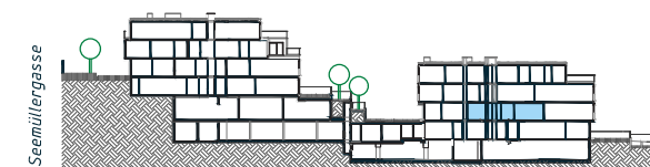
SCHNITT
